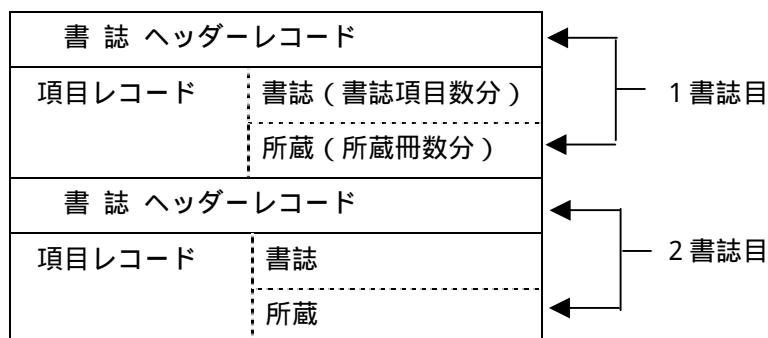
データ構造概略図
