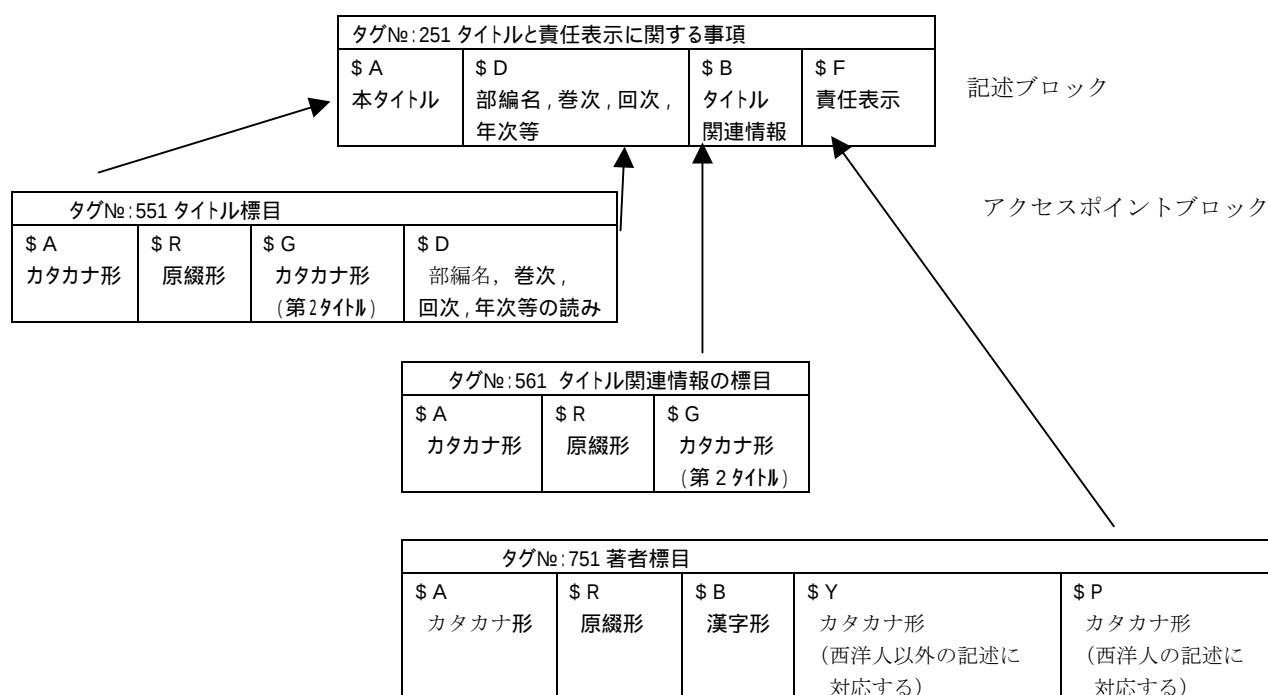
記述ブロックとアクセスポイントブロックの概念図
